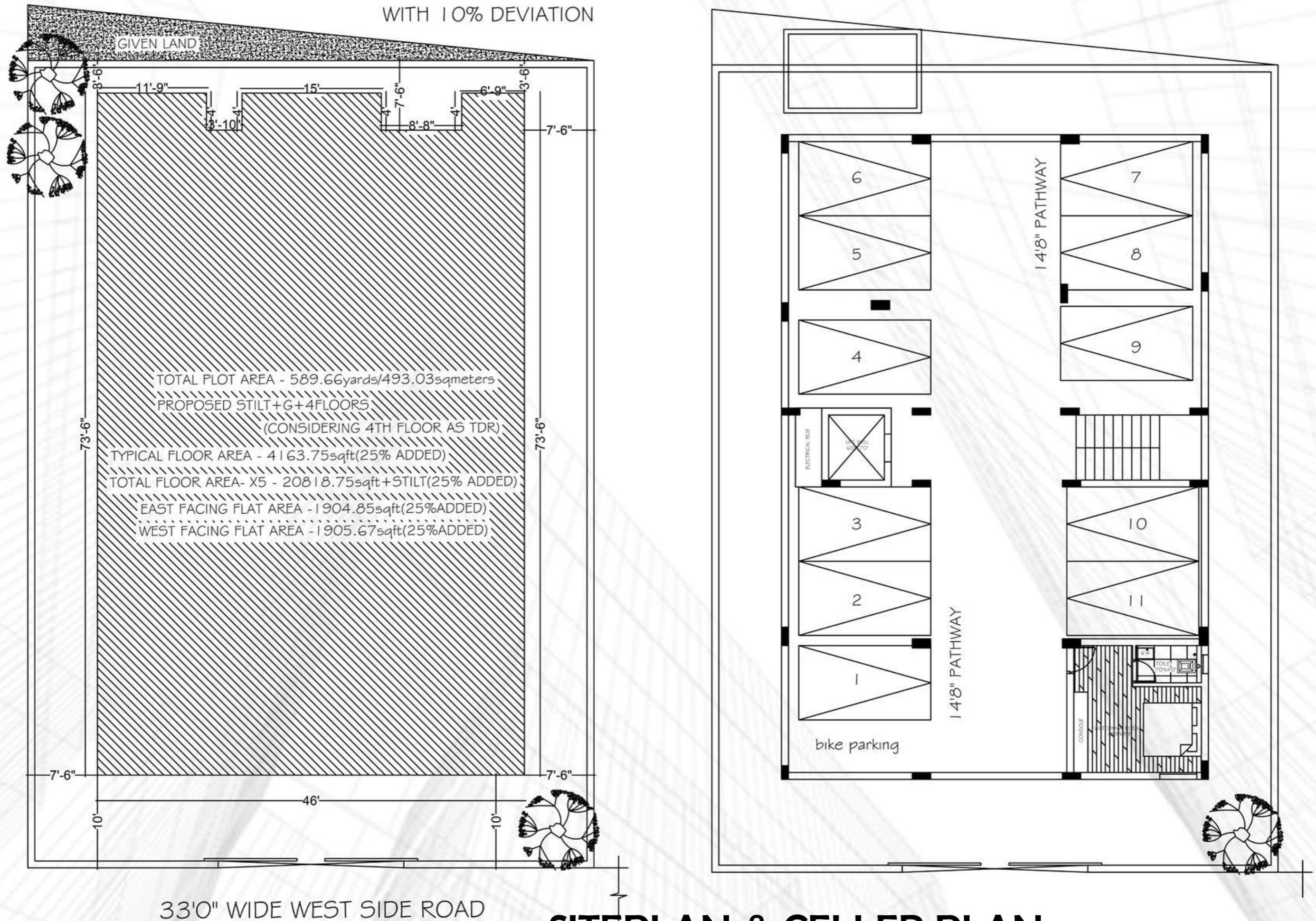
SITEPLAN & CELLER PLAN
